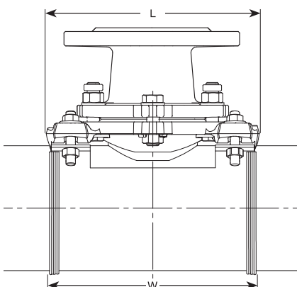
Хомут для ПЭ/ПВХ-О труб
